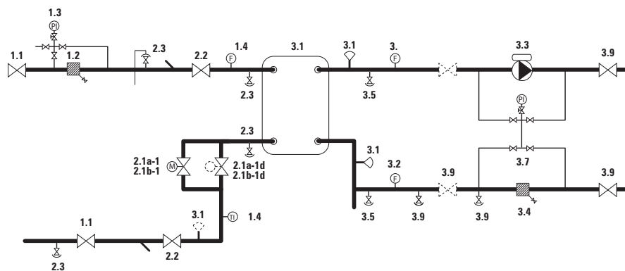
Kopplingschema
