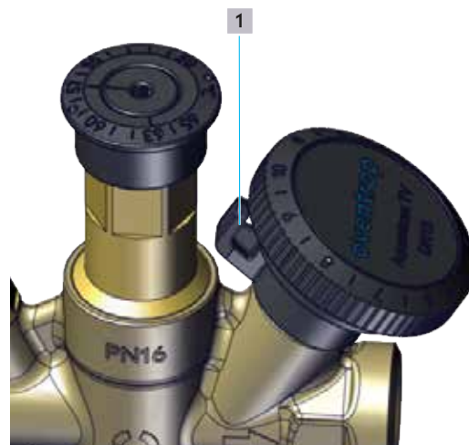
Fig. 11 - Preimpostazione
