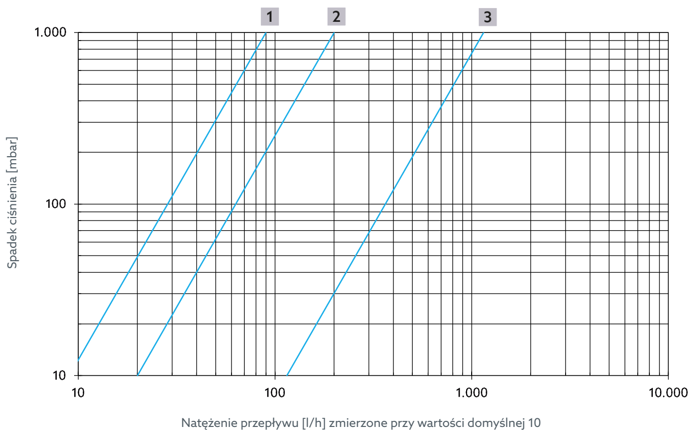
Ryc. 17: Natężenie przepływu regulacji termicznej dla artykułów numer 4202504, 4202604, 4202704, 4202804
