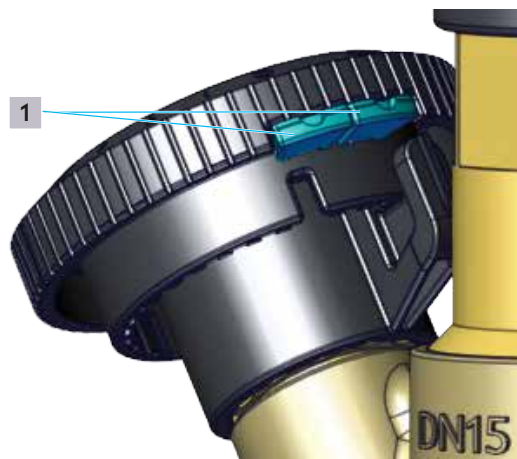
Abb. 12: Position Begrenzungsclips im Auslieferungszustand
