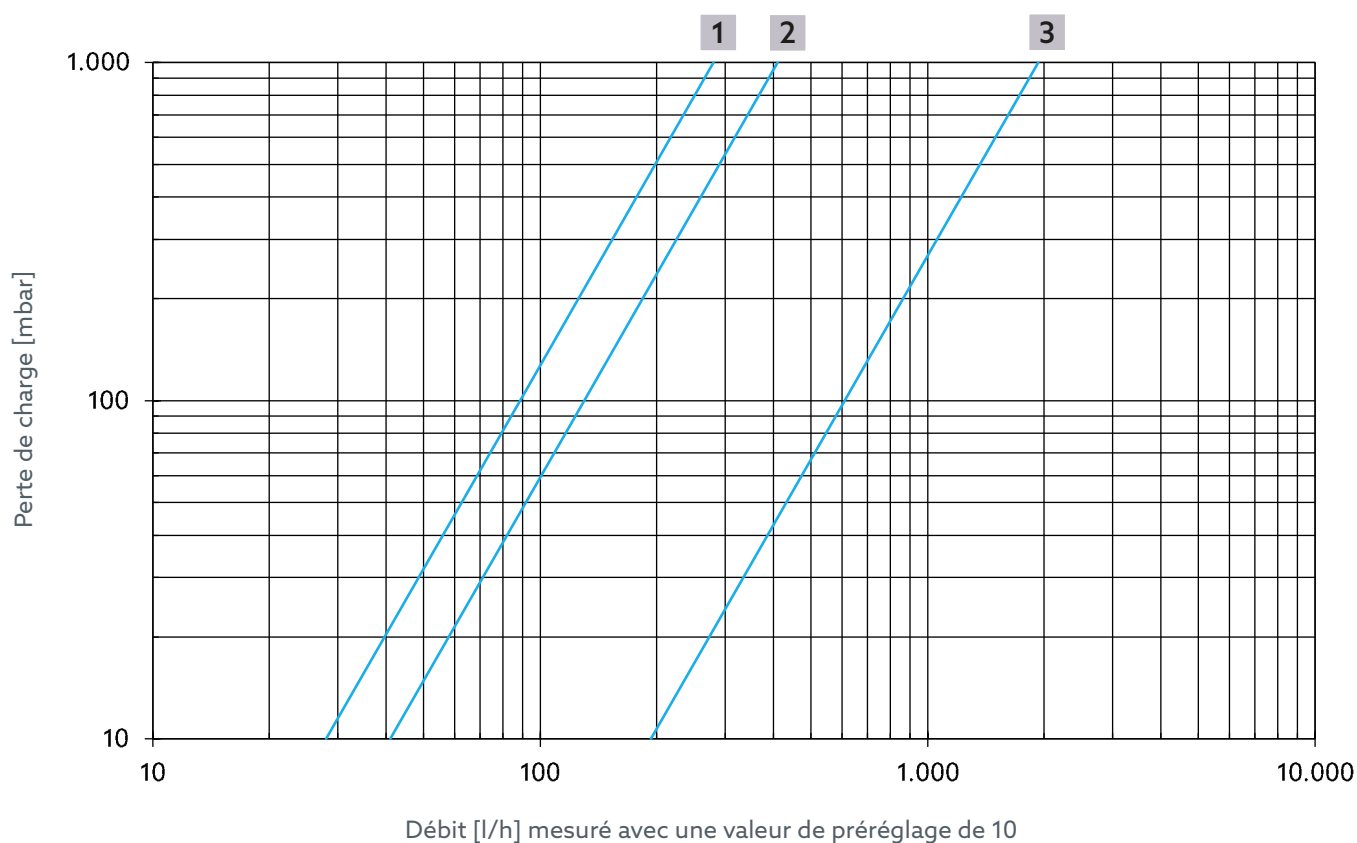
Fig. 19: Débit du réglage thermique pour réf. 4202506, 4202606, 4202706, 4202806
