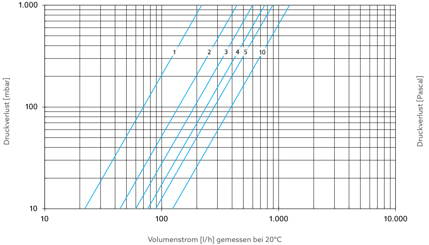
Abb. 15: Volumenstromvoreinstellung DN 15
