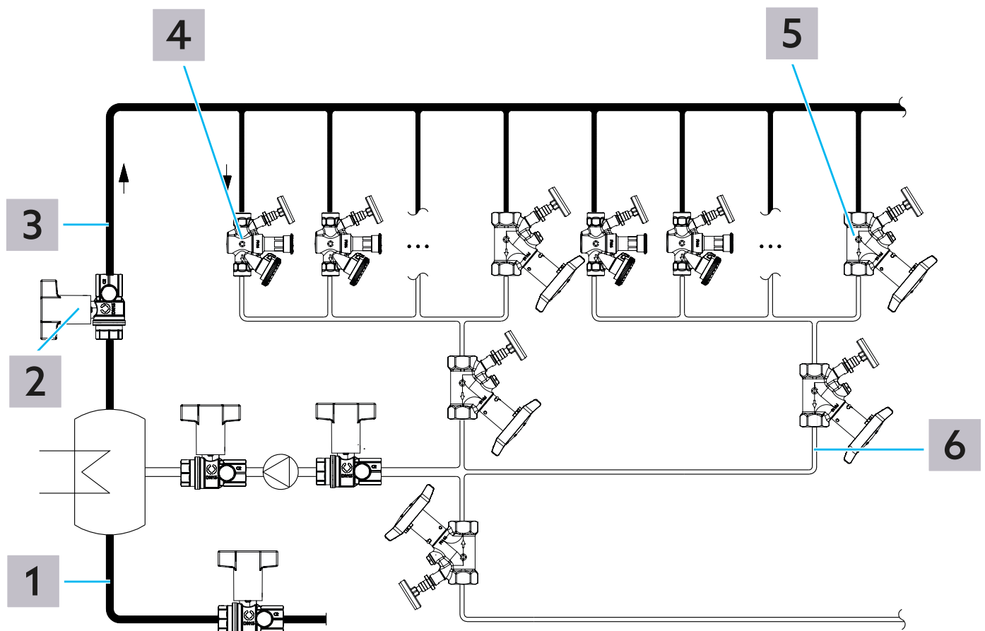
Obr. 4: Schéma zariadenia
