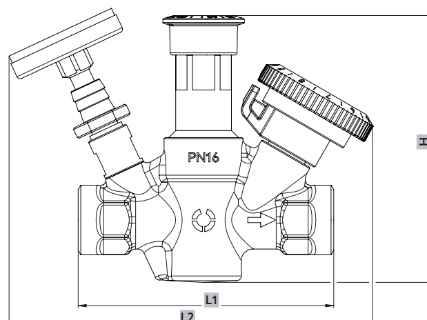
Fig. 2: Encombres latéraux
