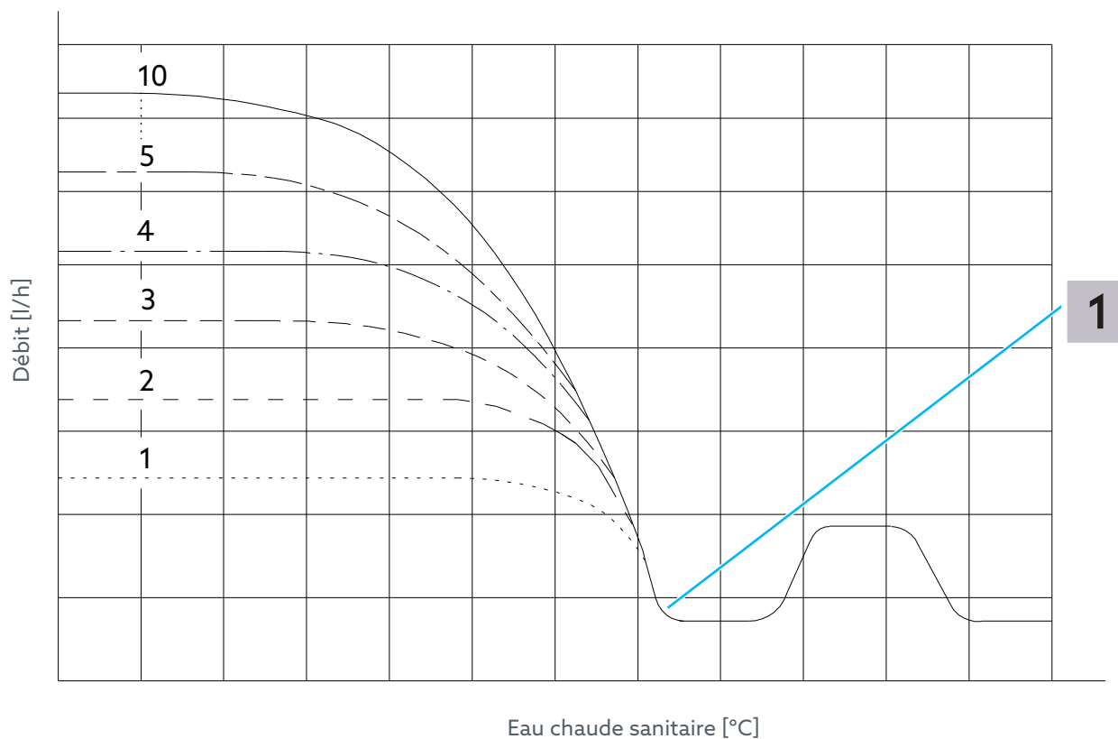
Fig. 7: Limitation du débit
