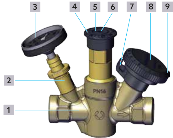
Fig. 1: Diseño
