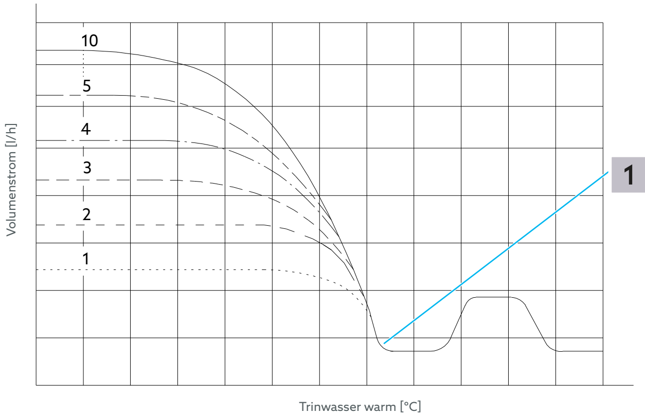
Abb. 7: Volumenstrombegrenzung
