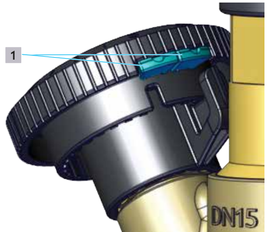
Fig. 12: Posición de los clips de límite en el estado de entrega
