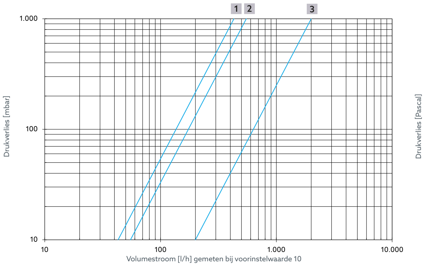
Afb. 20: Volumestroom Thermische regeling voor artikelnummers 4202554 en 4202754
