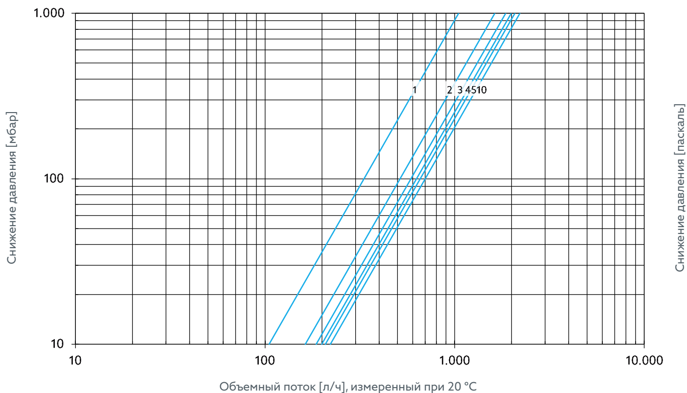
Рис. 16: Предварительная настройка объемного потока DN 20
