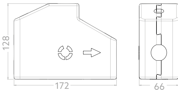
Abb. 5: Dämmschale
