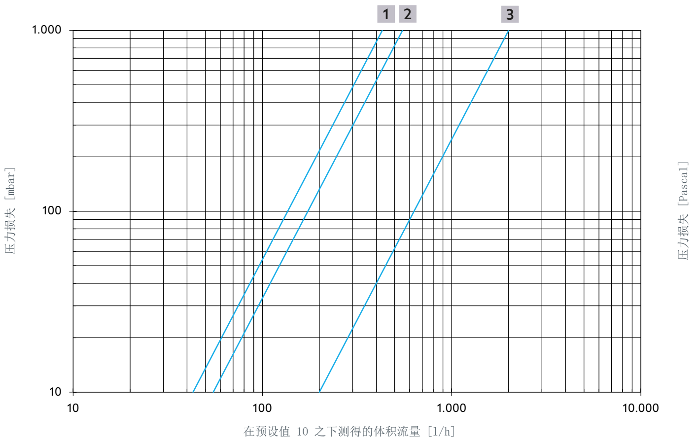
图 20: 产品编号 4202554 和 4202754 的体积流量热力调节
