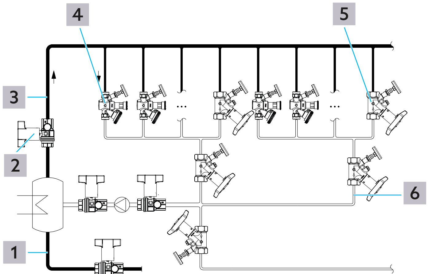
Abb. 4: Anlagenschema
