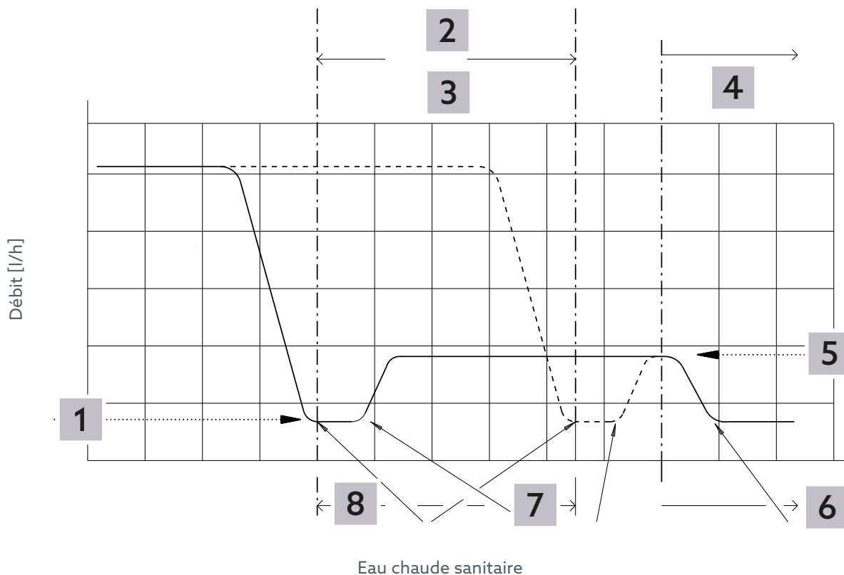
Fig. 6: Comportement de régulation thermique
