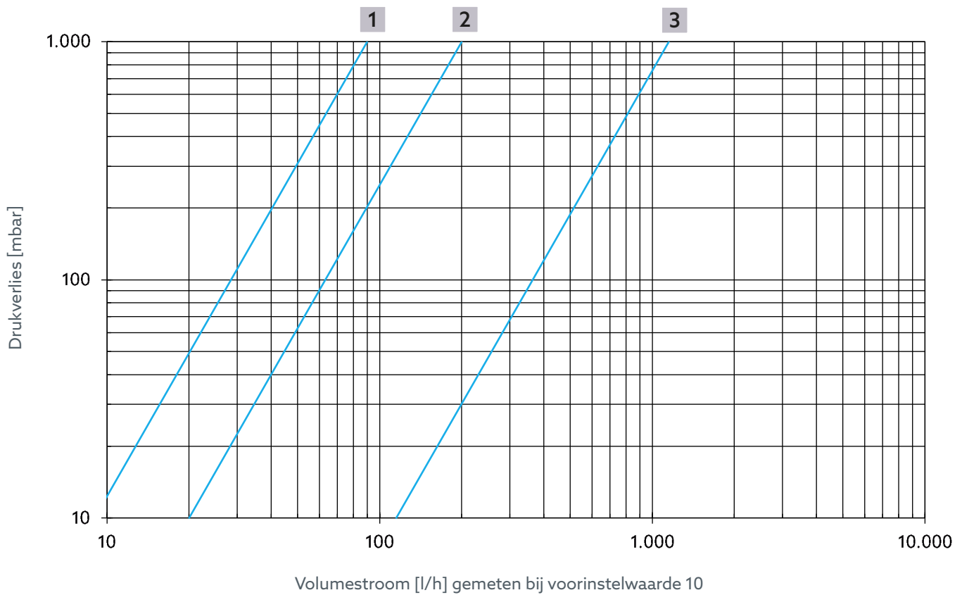
Afb. 17: Volumestroom Thermische regeling voor artikelnummers 4202504, 4202604, 4202704, 4202804
