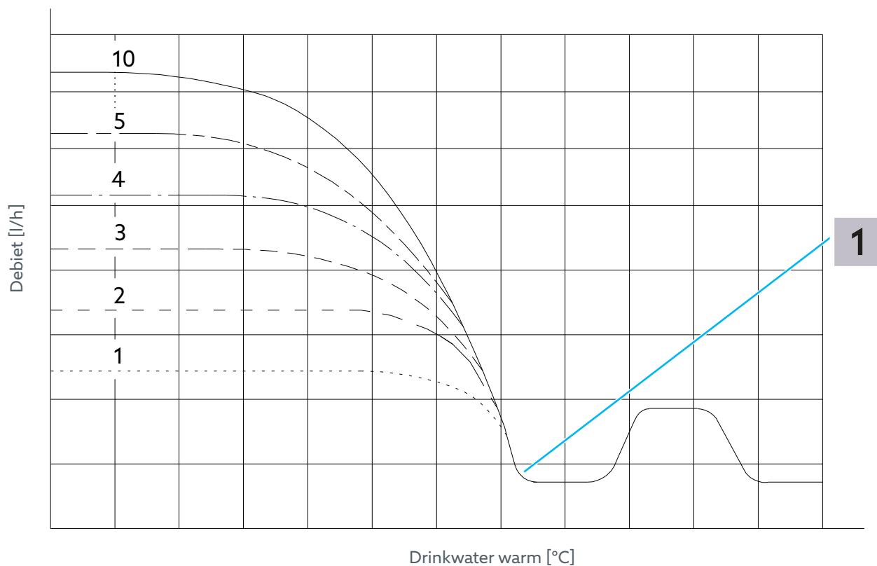
Afb. 7: Volumestroombegrenzing
