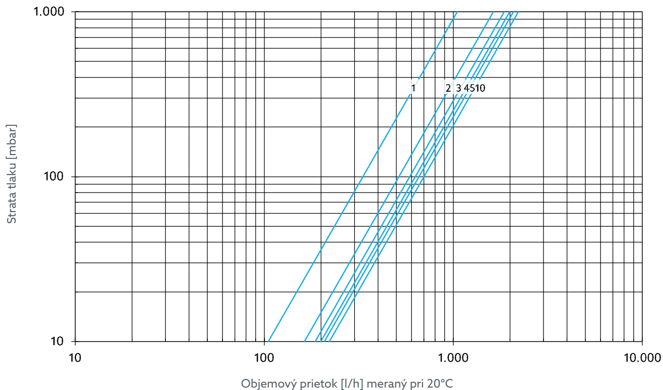
Obr. 16: Prednastavenie objemového prietoku DN 20
