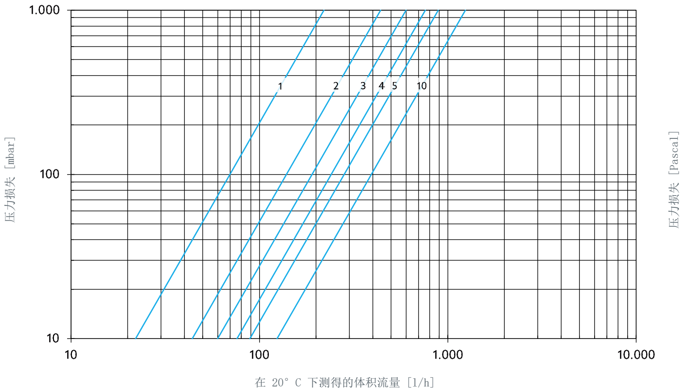
图 15: 体积流量预设置 DN 15
