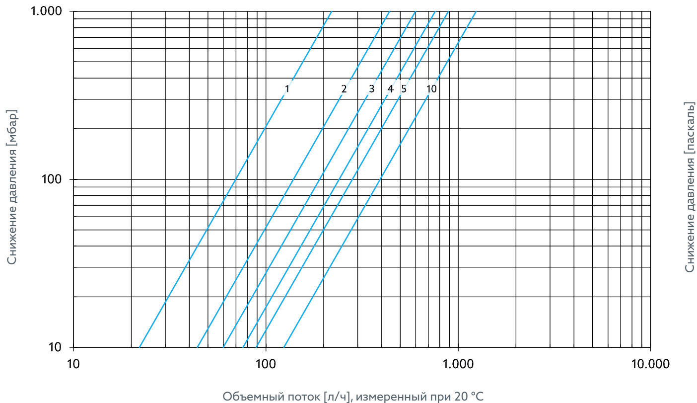
Рис. 15: Предварительная настройка объемного потока DN 15
