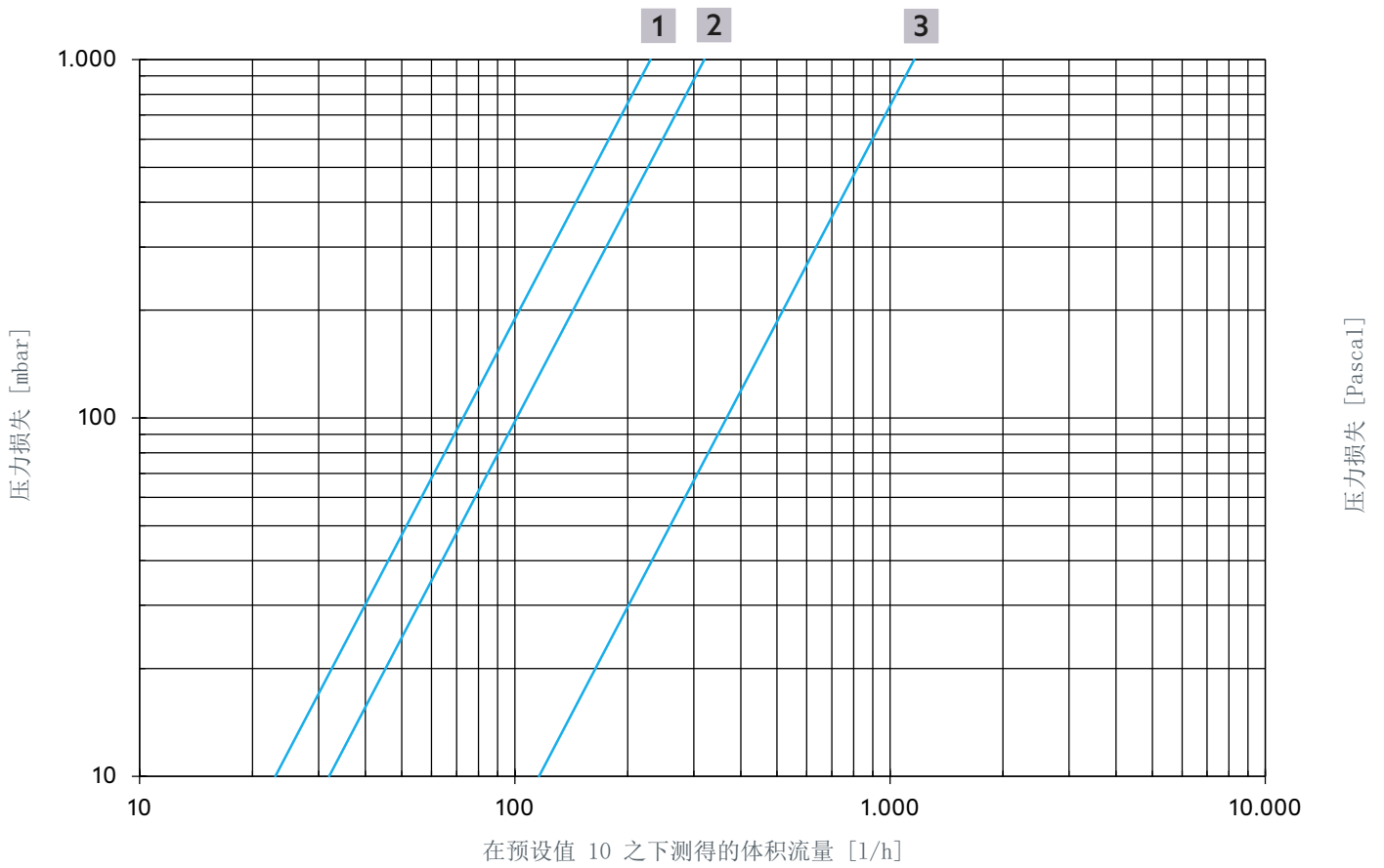
图 18: 产品编号 4202553 和 4202753 的体积流量热力调节
