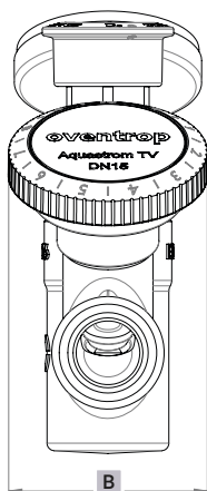
Fig. 3: Dimensiones frontales
