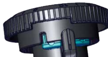
Abb. 14: Voreinstellung blockiert
