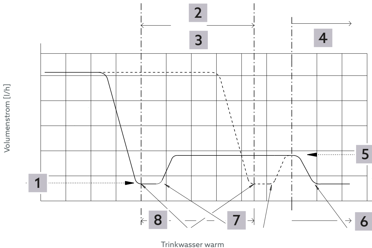
Abb. 6: Thermisches Regelverhalten
