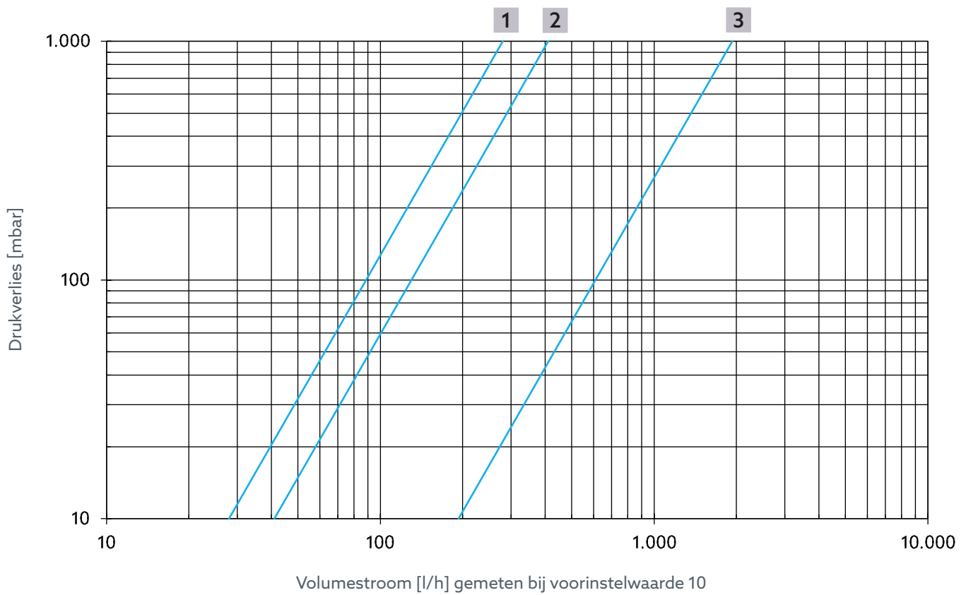
Afb. 19: Volumestroom Thermische regeling voor artikelnummers 4202506, 4202606, 4202706, 4202806
