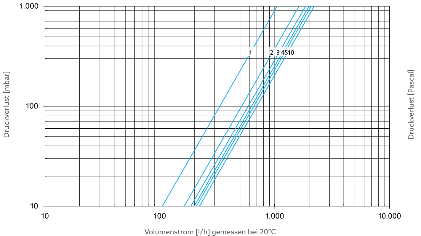
Abb. 16: Volumenstromvoreinstellung DN 20
