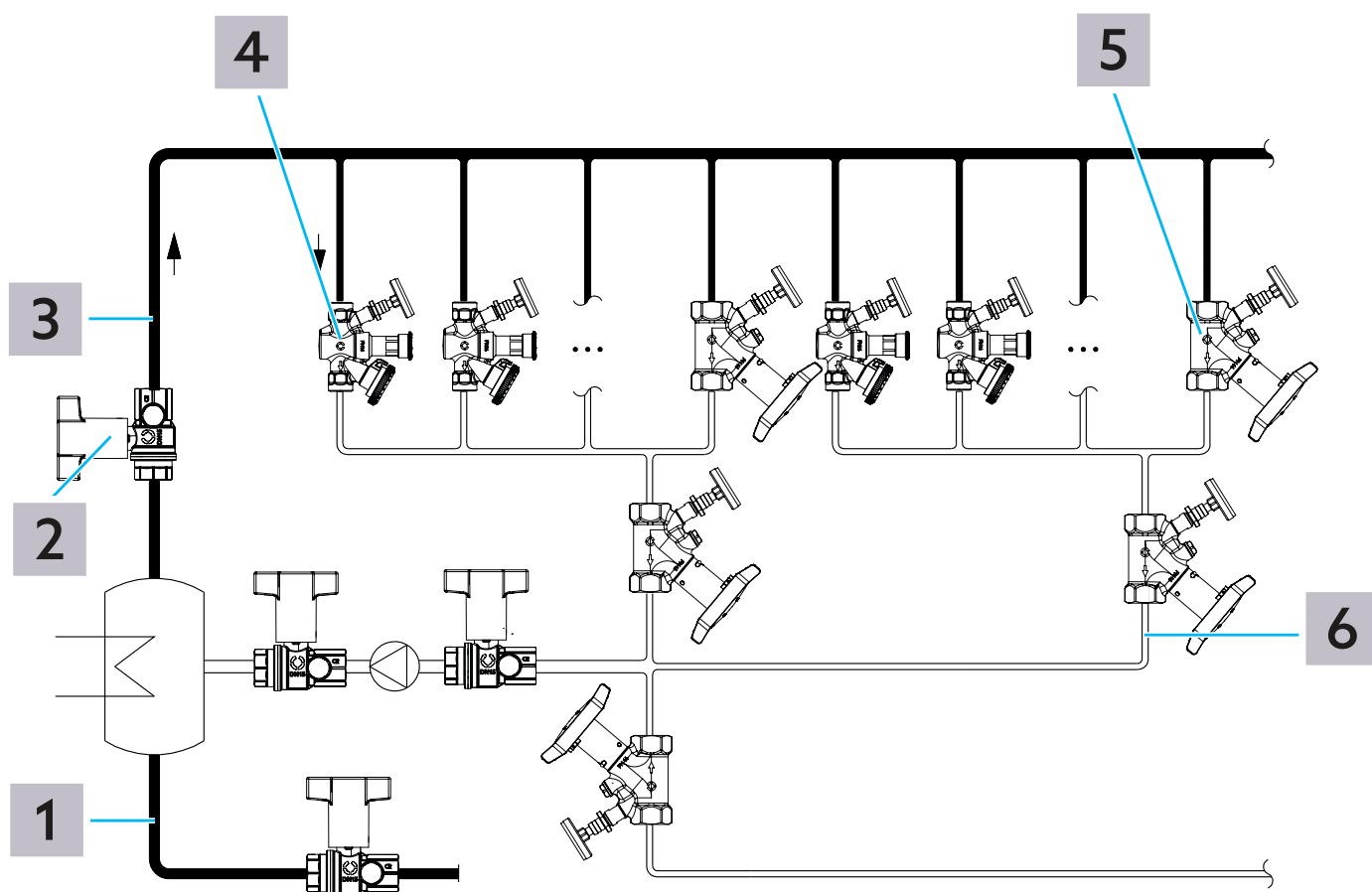
Fig. 4 - Schema dell'impianto
