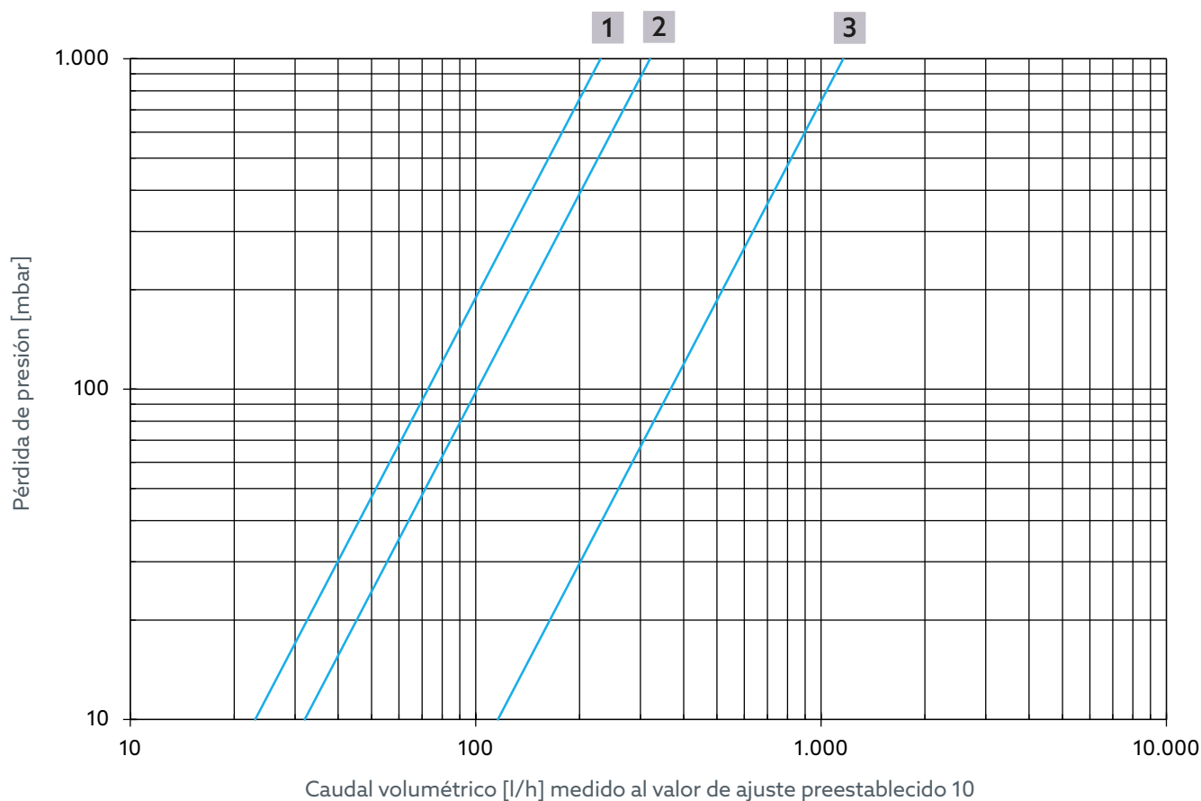
Fig. 18: Caudal volumétrico control térmico para los artículos n.º 4202553 y 4202753
