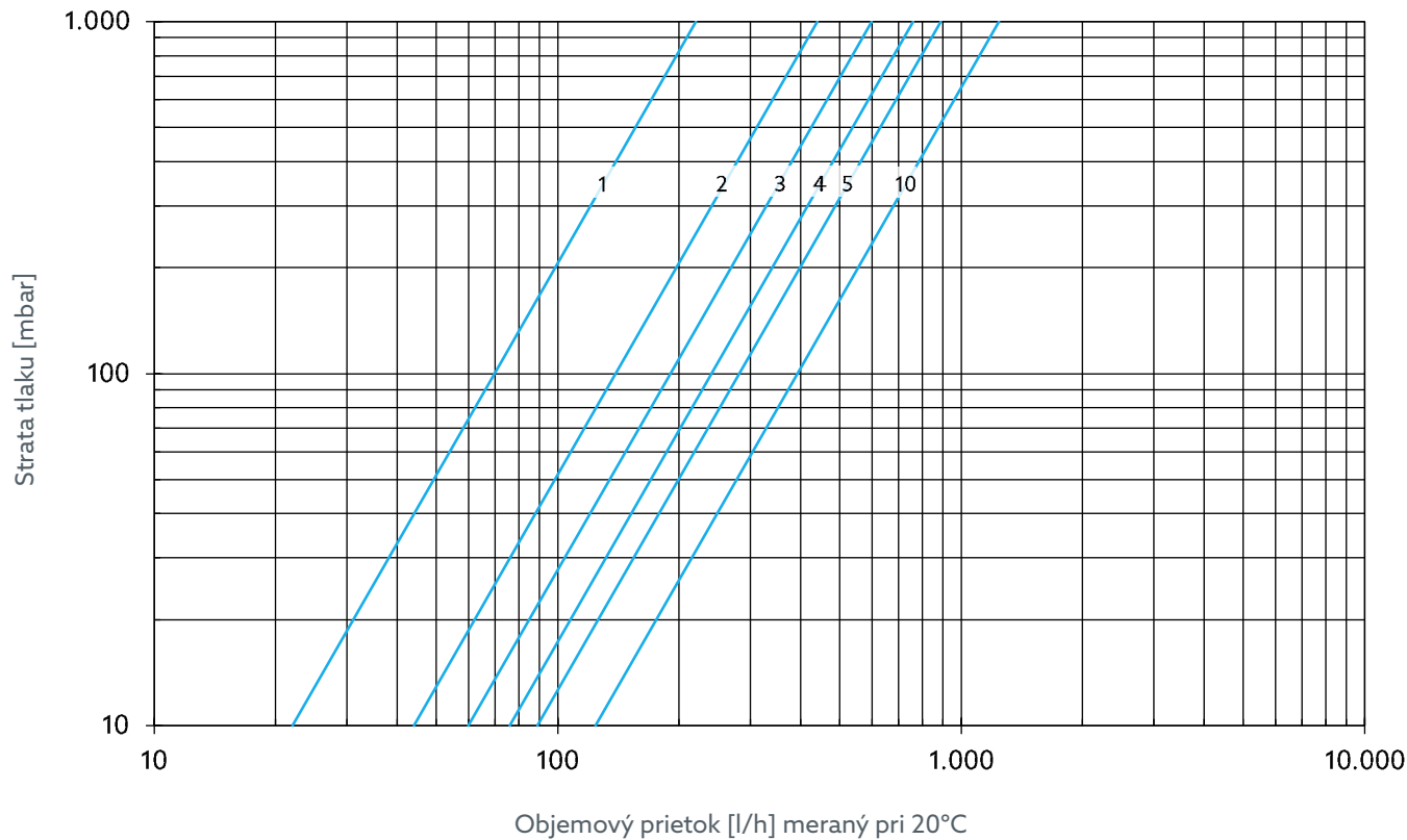
Obr. 15: Prednastavenie objemového prietoku DN 15
