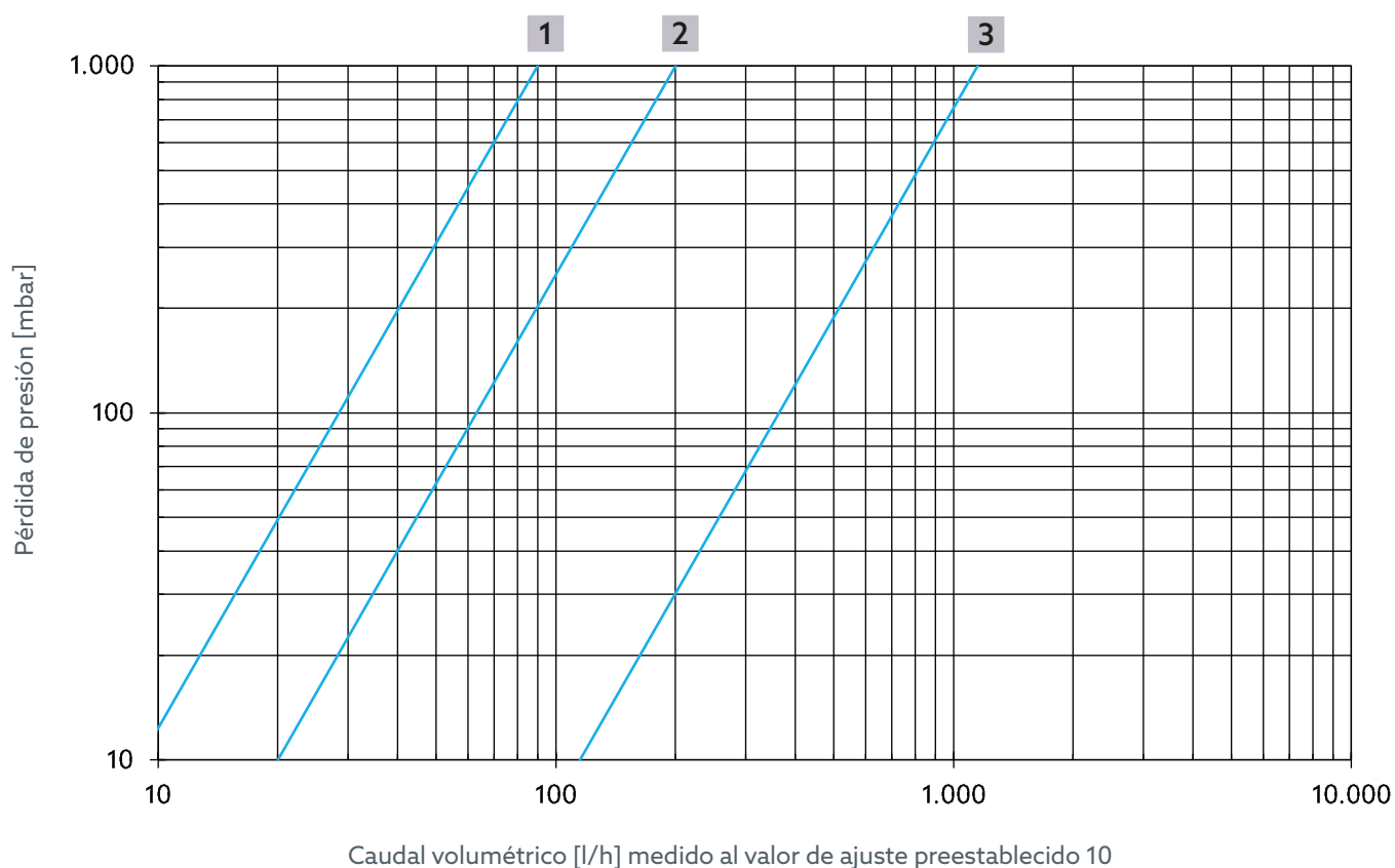
Fig. 17: Caudal volumétrico control térmico para los artículos n.º 4202504, 4202604, 4202704, 4202804
