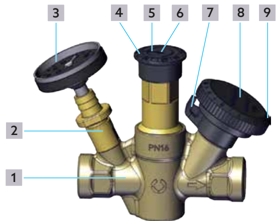
Afb. 1: Opbouw
