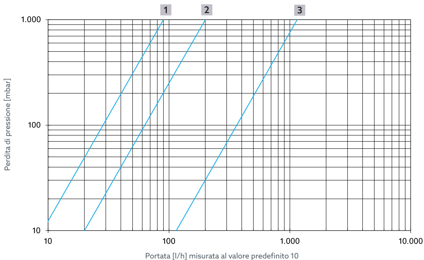
Fig. 17 - Portata regolazione termica dei codici articolo 4202504, 4202604, 4202704, 4202804
