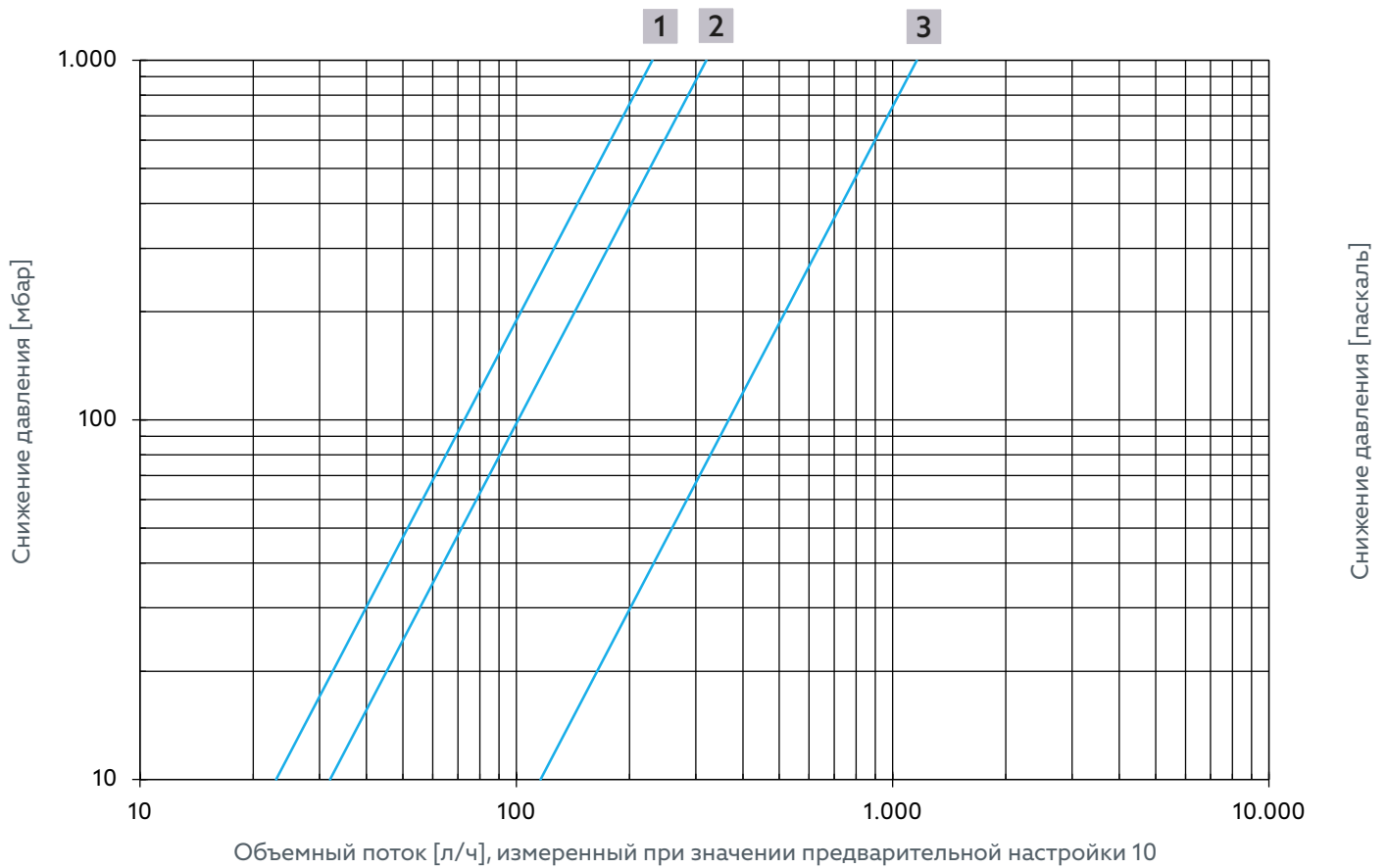
Рис. 18: Объемный поток Термическое регулирование для арт. № 4202506, 4202606, 4202706, 4202806
