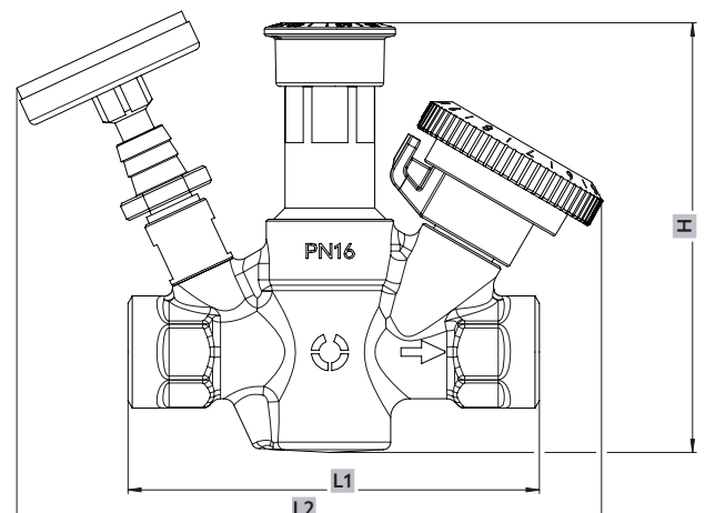
Fig. 2: Dimensiones laterales
