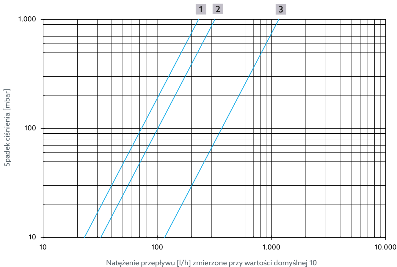
Ryc. 18: Natężenie przepływu regulacji termicznej dla artykułów numer 4202553 i 4202753
