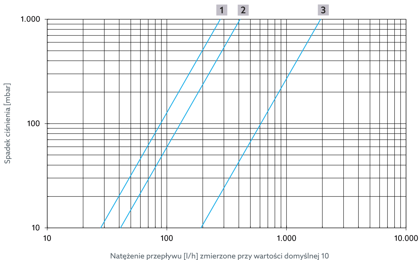
Ryc. 19: Natężenie przepływu regulacji termicznej dla artykułów numer 4202506, 4202606, 4202706, 4202806
