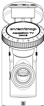
Abb. 3: Abmessungen frontal
