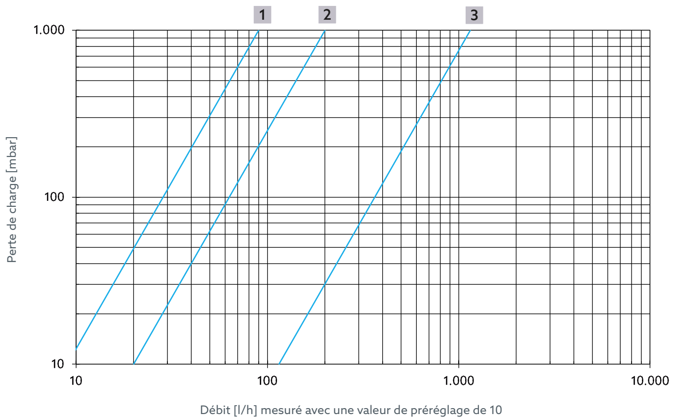
Fig. 17: Débit du réglage thermique pour réf. 4202504, 4202604, 4202704, 4202804
