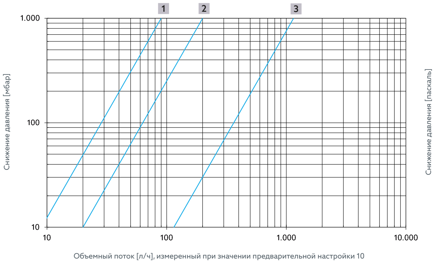
Рис. 17: Объемный поток Термическое регулирование для арт. № 4202504, 4202604, 4202704, 4202804
