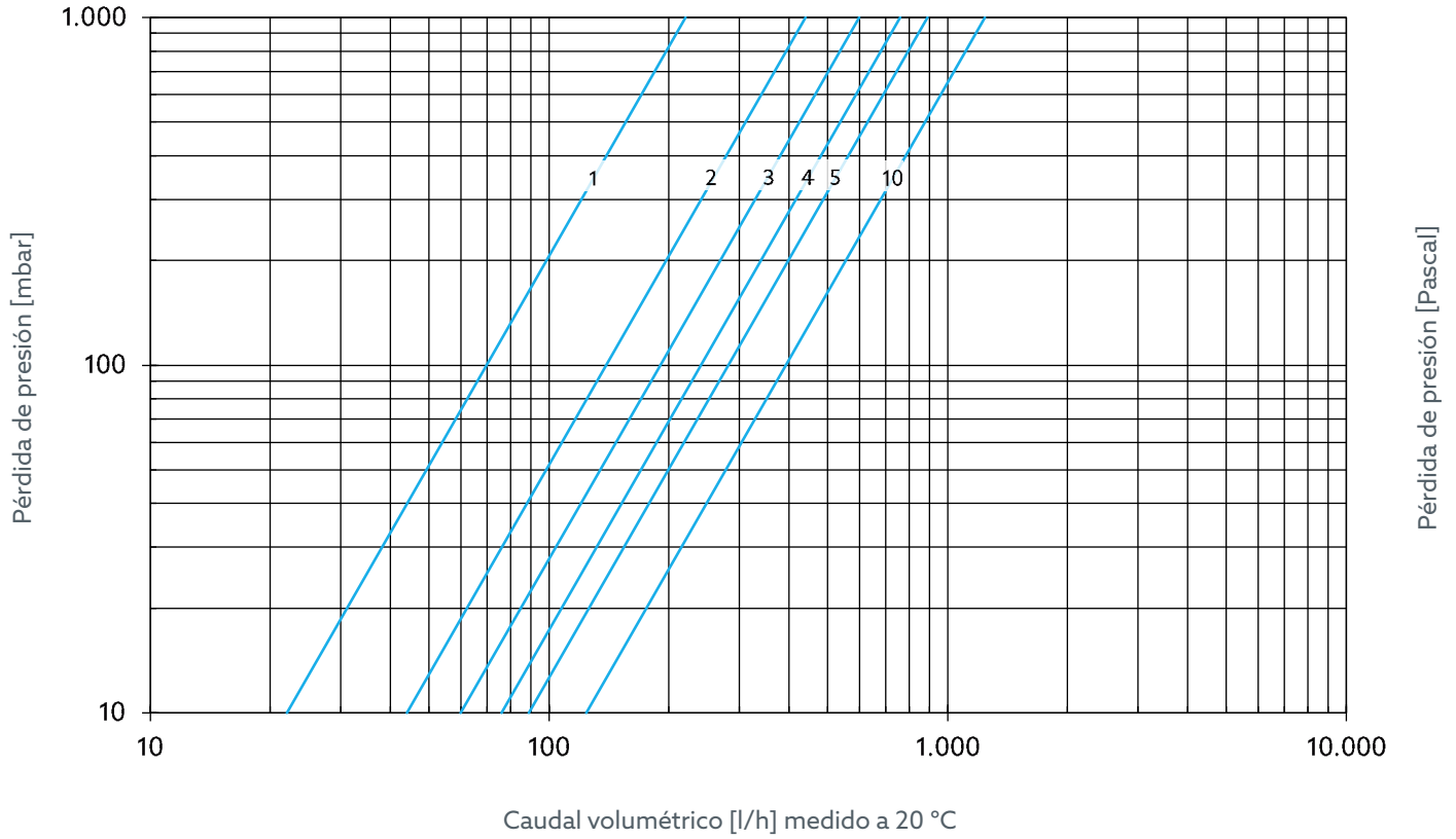
Fig. 15: Caudal volumétrico preestablecido DN 15
